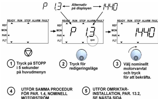
Figur 2: Vacon 10 startguide (program för allmän användning)
